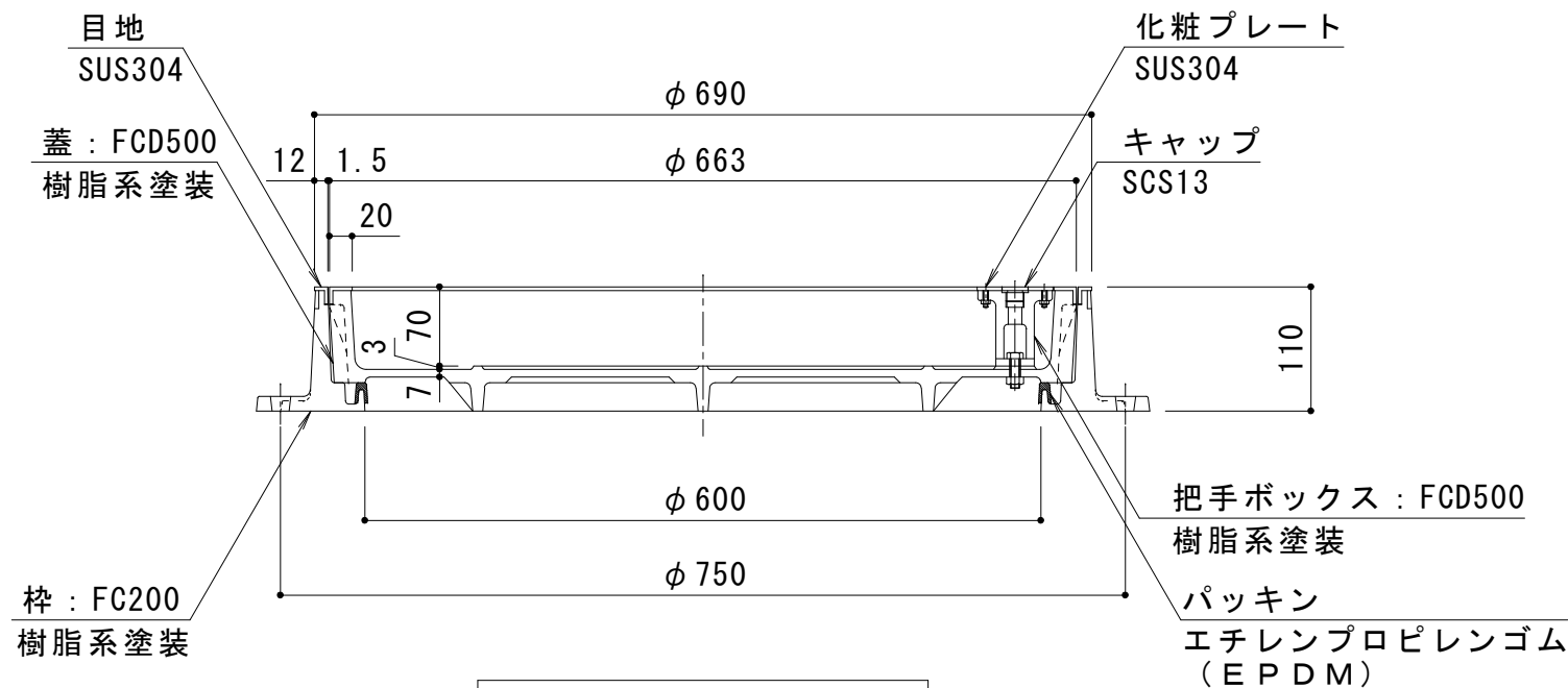
A-A断面図 S=1:7
