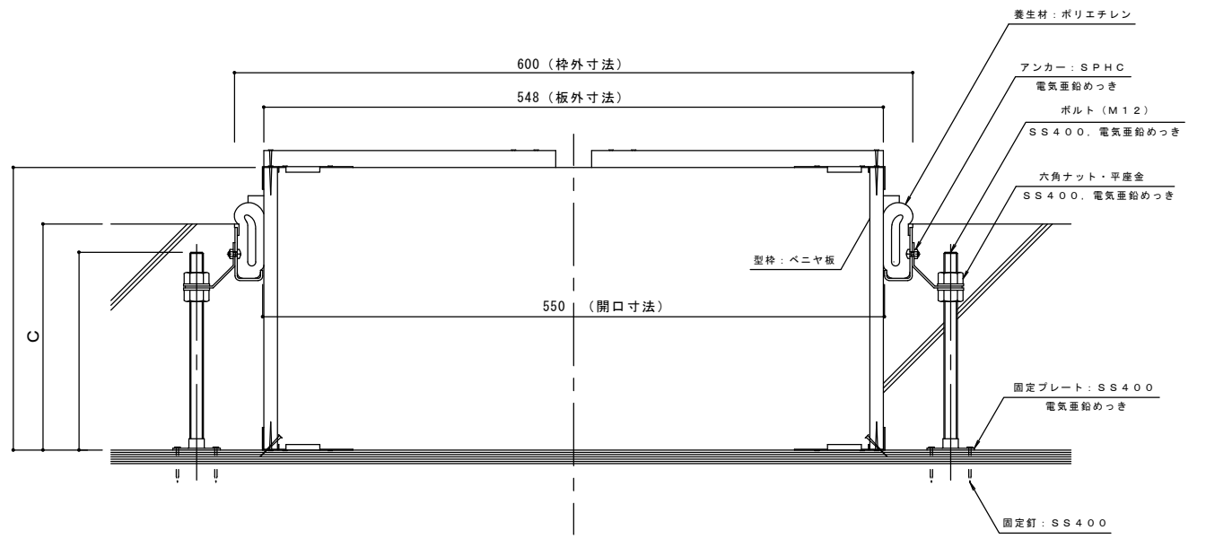
打込型フローハッチ RSV-1 (MSST-600-樹脂タイル貼物用-b) C= S=1:3
