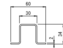
補強材詳細図 S=1:2
