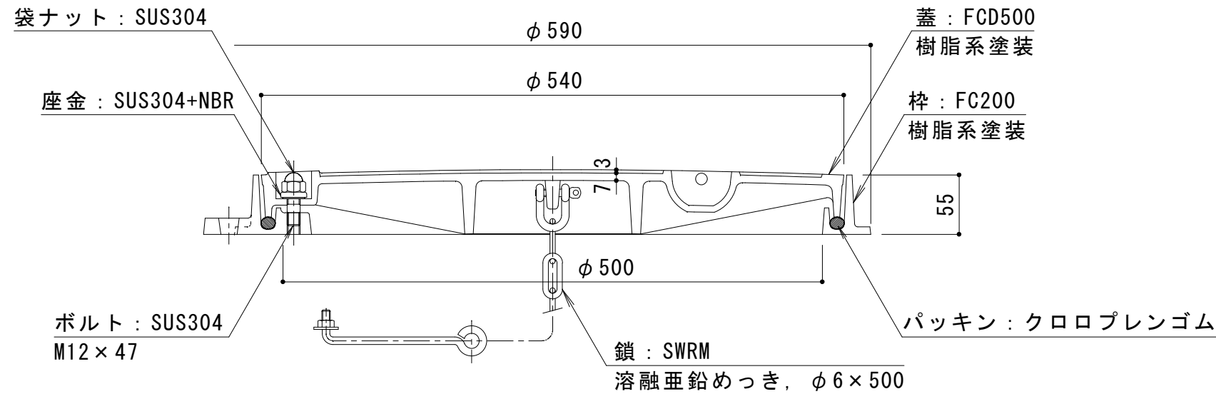
A-A 断面図
