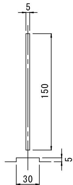
スリット部詳細 (120度振分けで3ヶ所)
