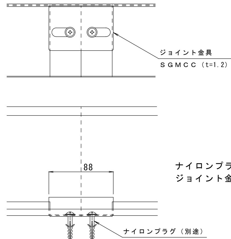
ジョイント金具取付納まり詳細図 S=1:3
