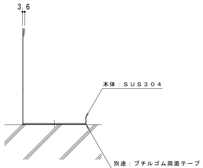
本体納まり断面詳細図 S=1:3
