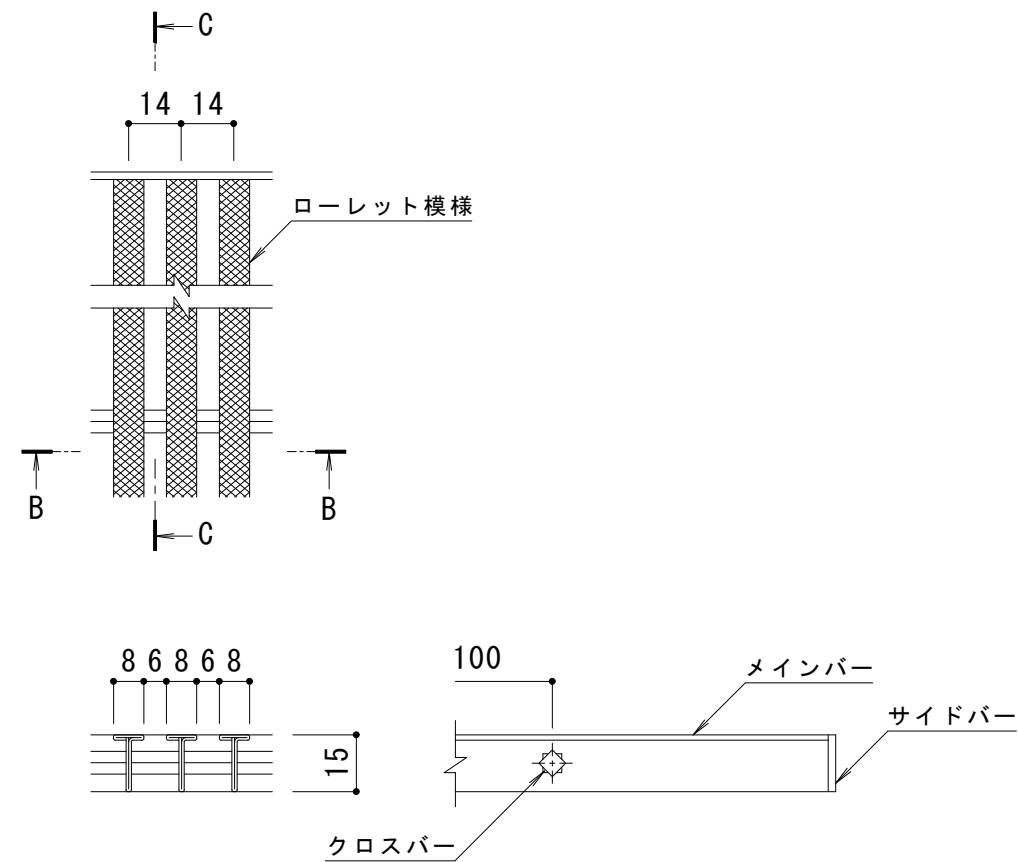
B-B断面図
