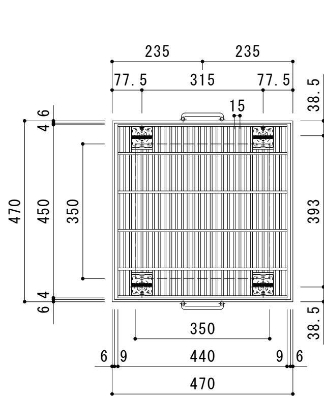
平面詳細図 S = 1 : 10
