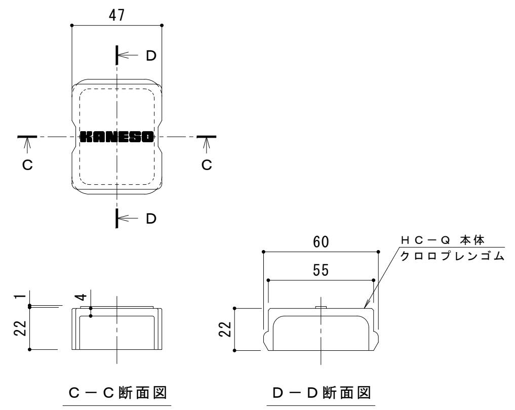
ボルトキャップ H C - Q 詳細図
