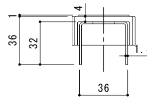
C-C断面図
