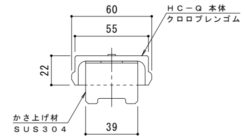
D-D断面図
