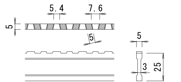
DI-25 バー形状詳細 S=1:2
