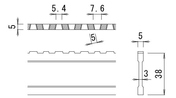
DI-38 バー形状詳細 S=1:2
