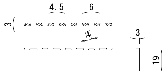
DFB3×19 バー形状詳細 S=1:2
