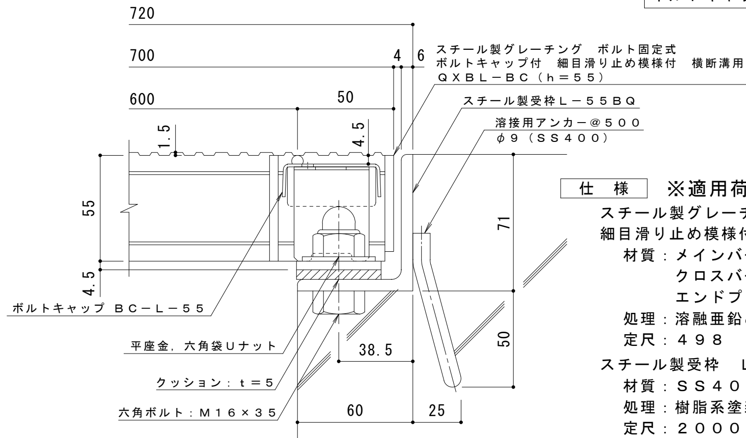
ボルトキャップBC-L詳細図
