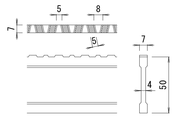
DI-50 バー形状詳細 S=1:2
