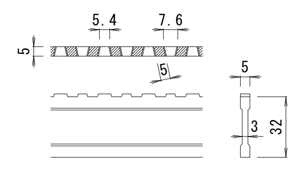
DI-32 バー形状詳細 S=1:2
