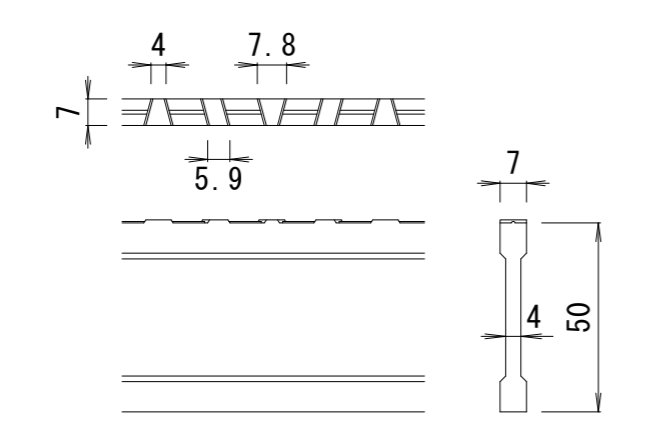
NSI-50 バー形状詳細 S = 1 : 2
