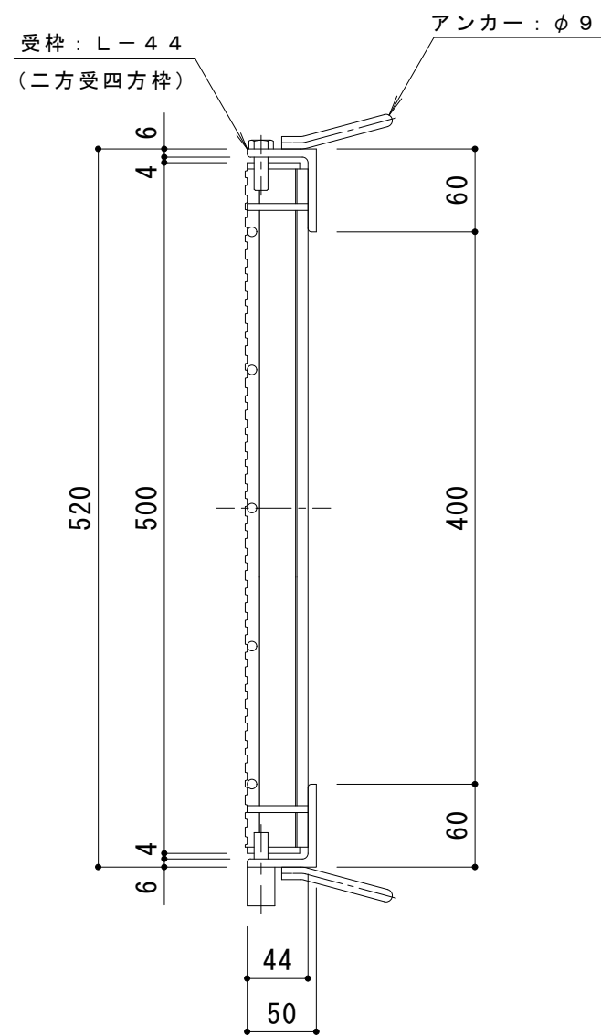
DI-44 バー形状詳細 S=1:2
