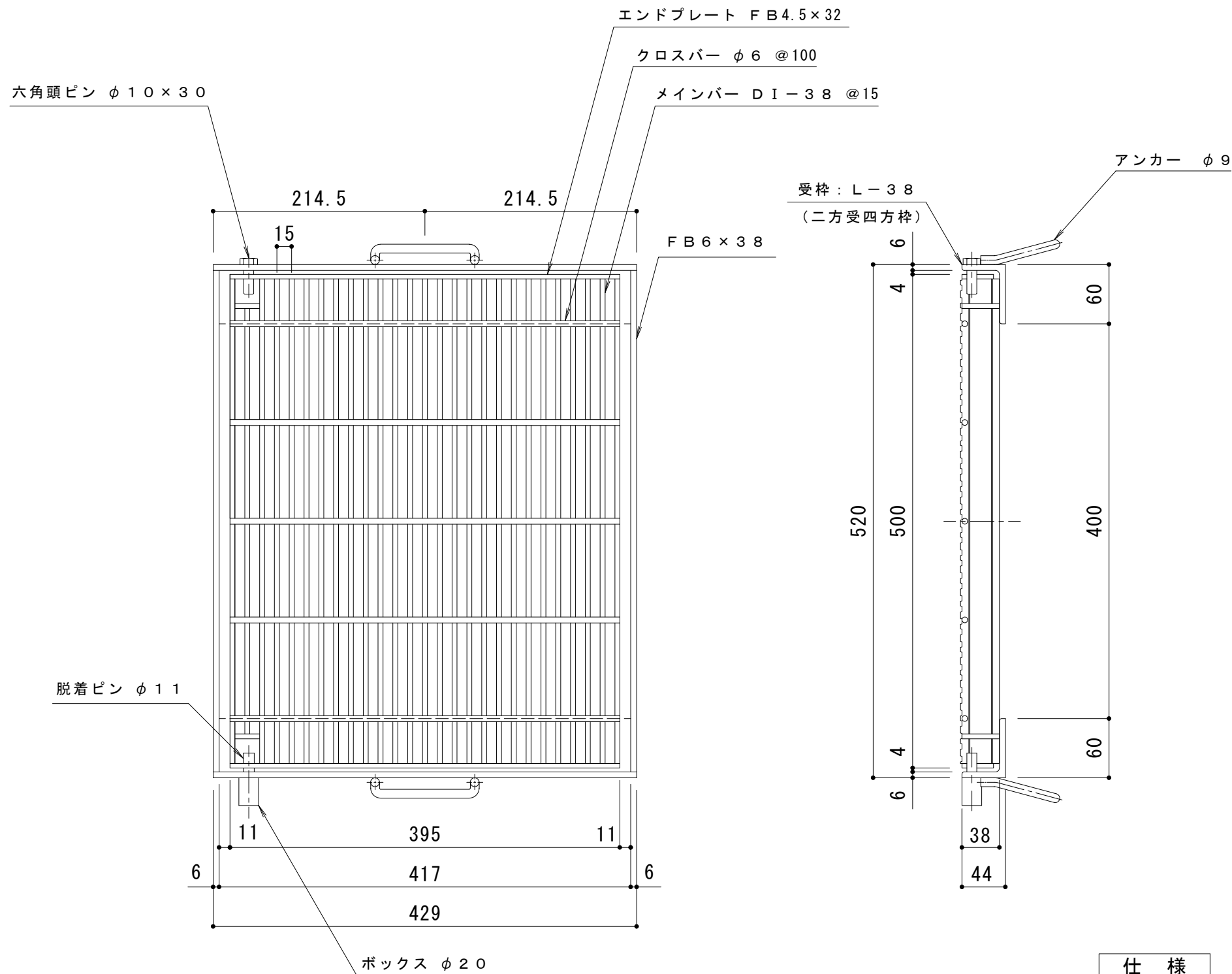
DI-38 バー形状詳細 S=1:2
