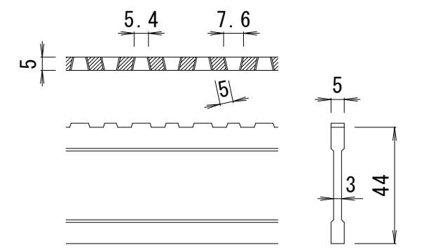
DI-44 バー形状詳細 S=1:2
