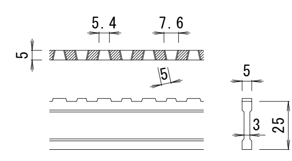
DI-25 バー形状詳細 S=1:2
