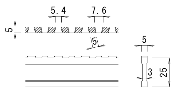
DI-25 バー形状詳細 S=1:2
