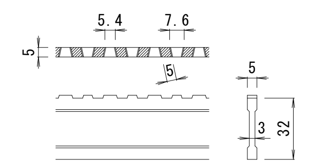
DI-32 バー形状詳細 S=1:2
