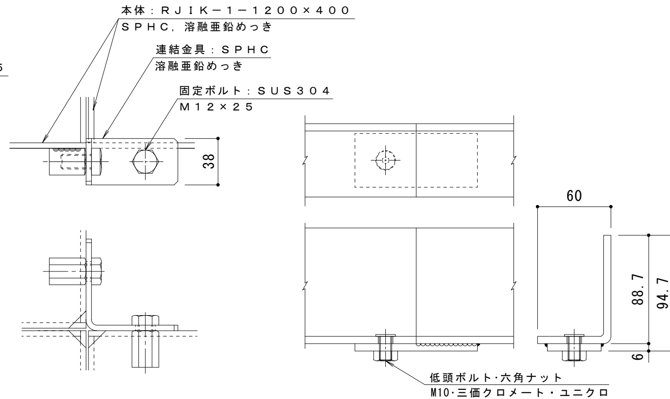
本体連結部詳細 S = 1 : 3 ※本体は8分割です。
