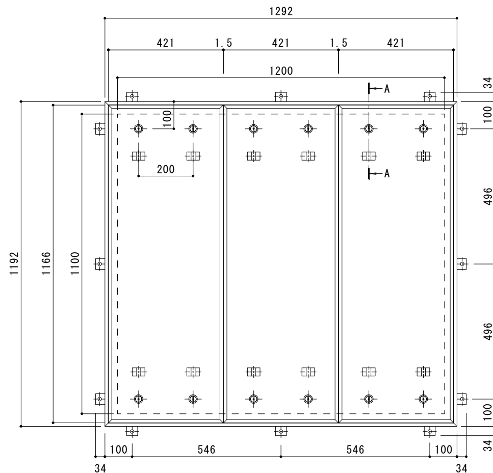
平面詳細図 S = 1 : 10
