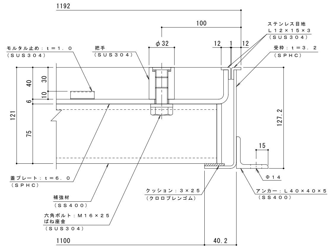
A-A断面詳細図 S = 1 : 2
