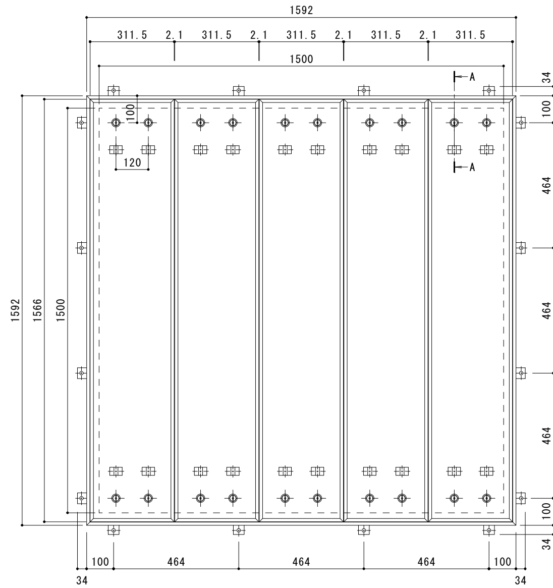
平面詳細図 S = 1 : 10
