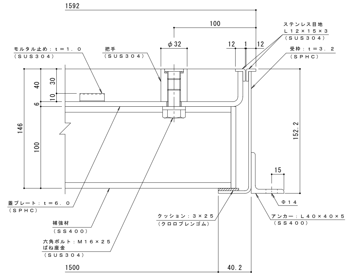
A-A断面詳細図 S = 1 : 2
