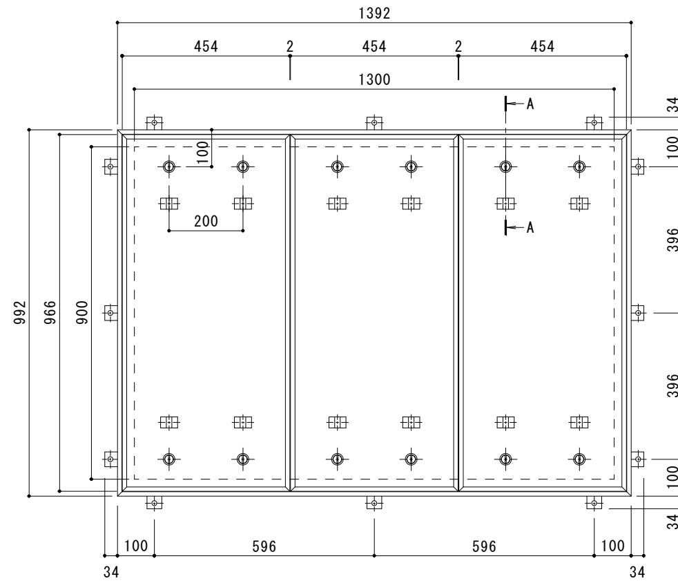
平面詳細図 S = 1 : 10
