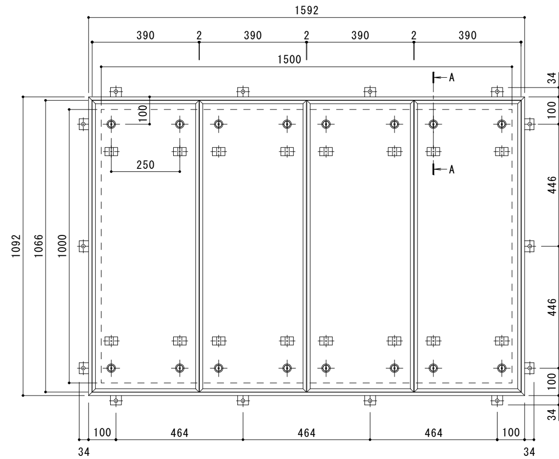
平面詳細図 S = 1 : 10
