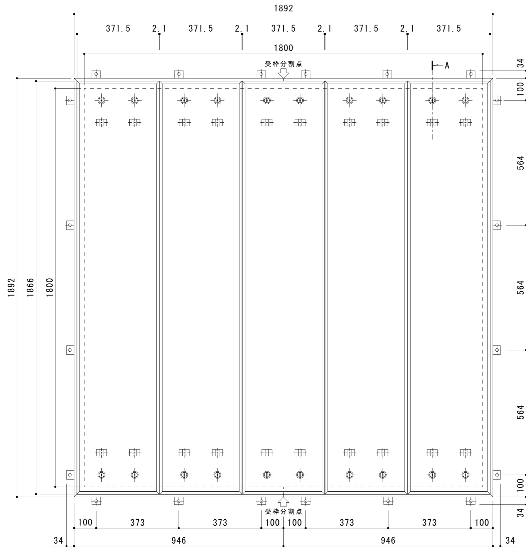
平面詳細図 S = 1 : 10
