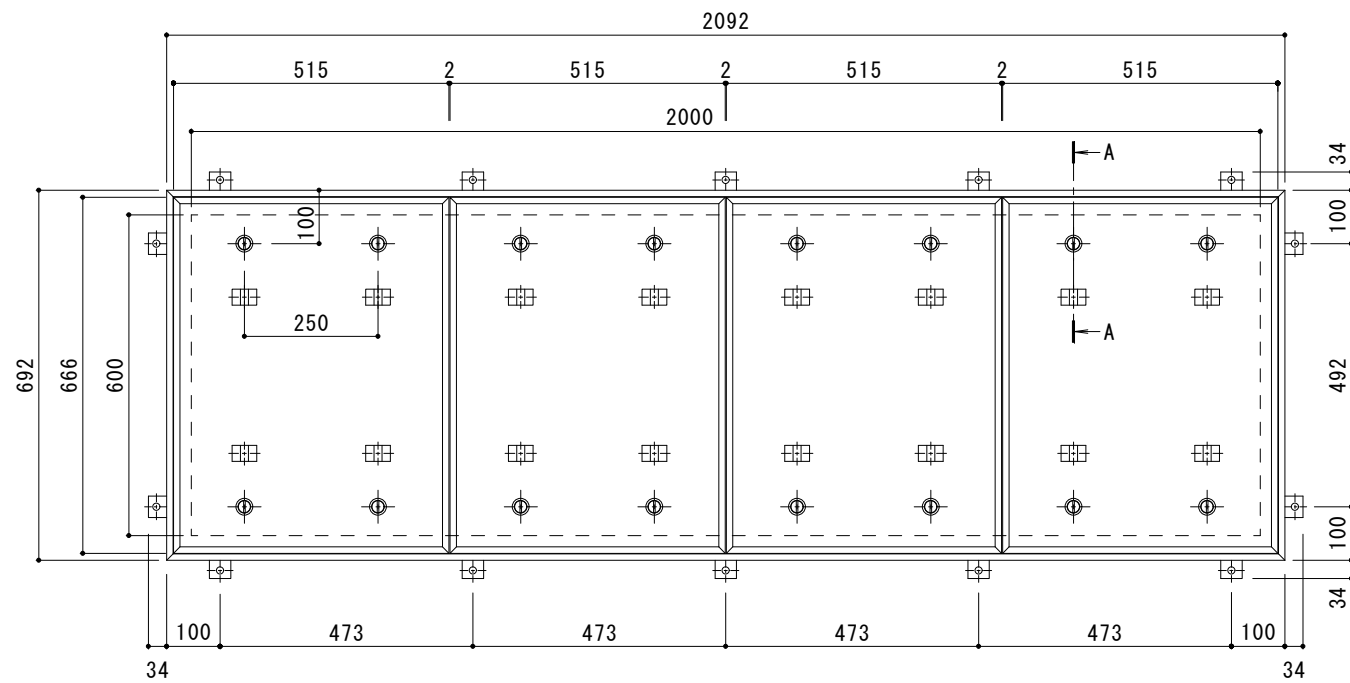
平面詳細図 S = 1 : 10
