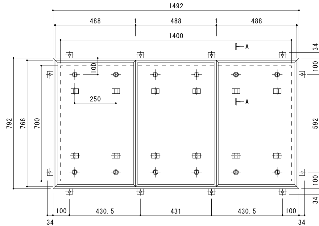
平面詳細図 S = 1 : 10
