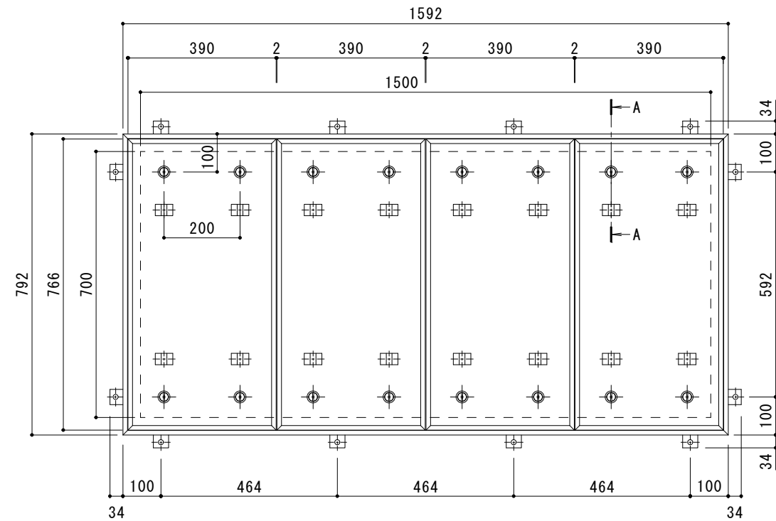
平面詳細図 S = 1 : 10
