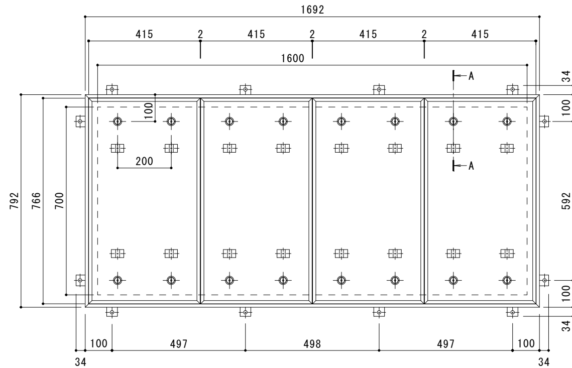
平面詳細図 S = 1 : 10
