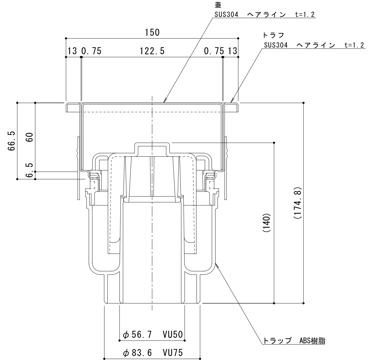
断面詳細図 S = 1 : 2
