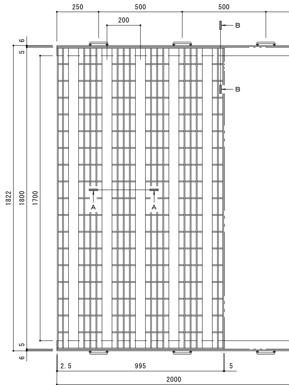
平面図 S = 1 : 10
