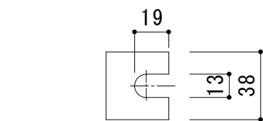
断面詳細図 S = 1 : 3
