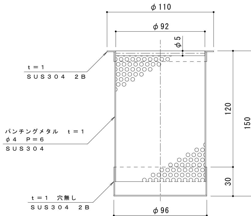
バスケット詳細図
