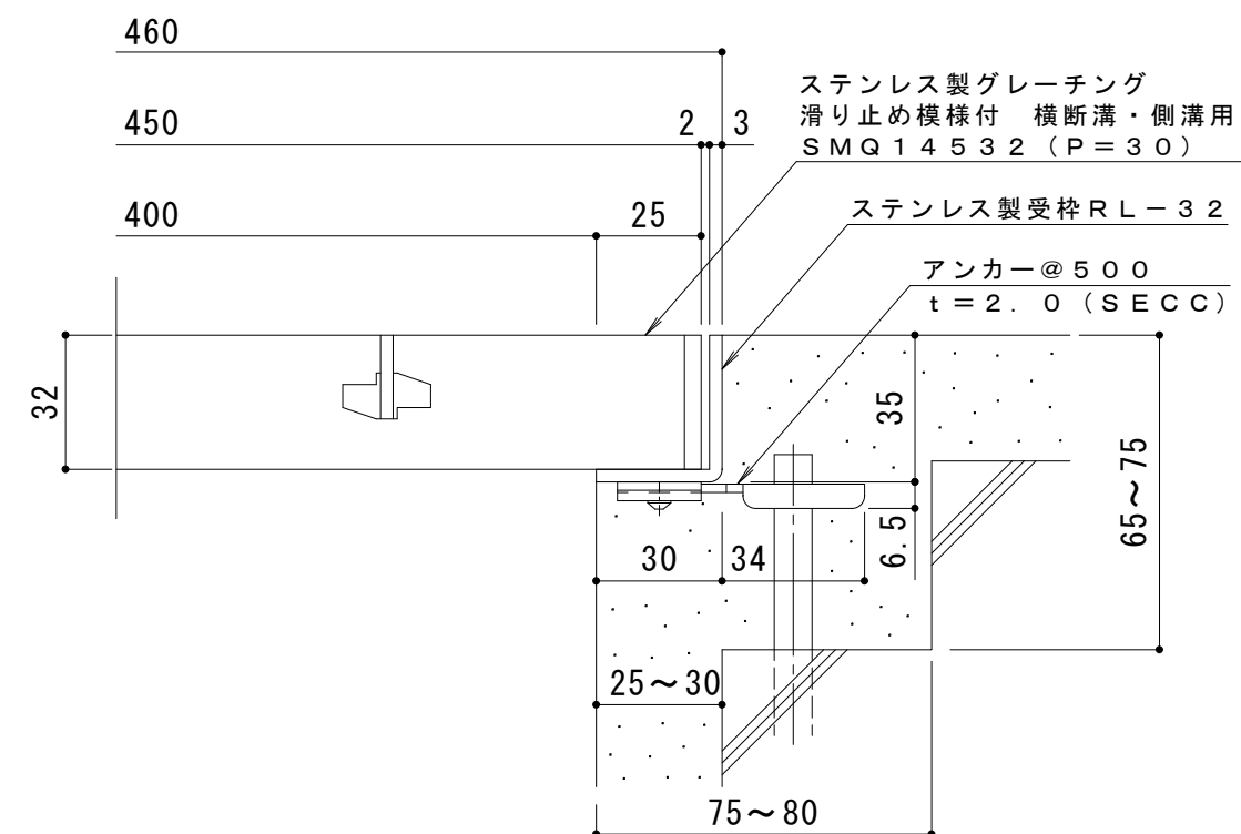
※適用荷重：歩行用（横断溝用） 仕 様 ※適用荷重：T-2（側溝用） ステンレス製グレーチング 滑り止め模様付 横断溝・側溝用 SMQ 1 4 5 3 2 （P=30） 材質：メインバー FB4×32（SUS304） クロスバー FB3×20（SUS304） サイドバー FB4×32（SUS304） 定尺：994 ステンレス製受枠 RL-32 材質：ステンレス鋼板 t=3.0（SUS304） 定尺：2000 施工場所の状況に合わせて、アンカーをプライヤー等で折り
