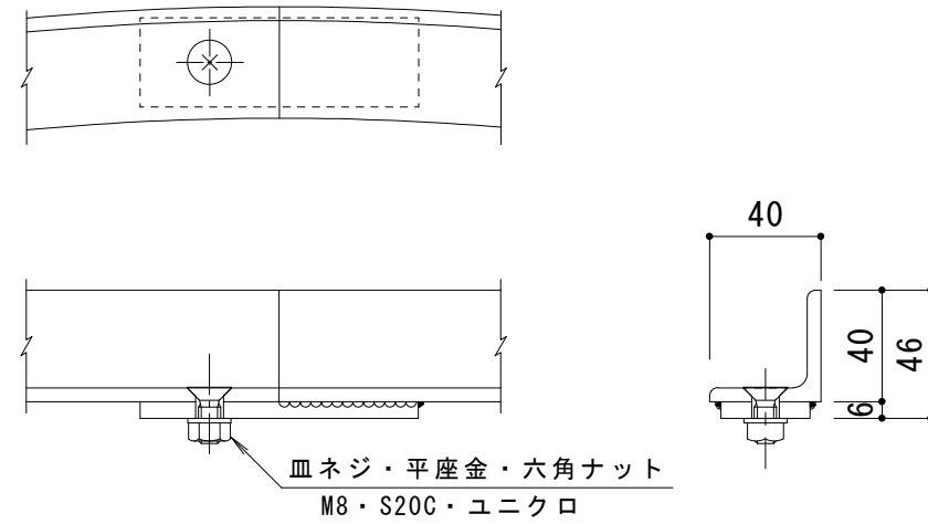
接続部詳細図 S = 1 : 3
