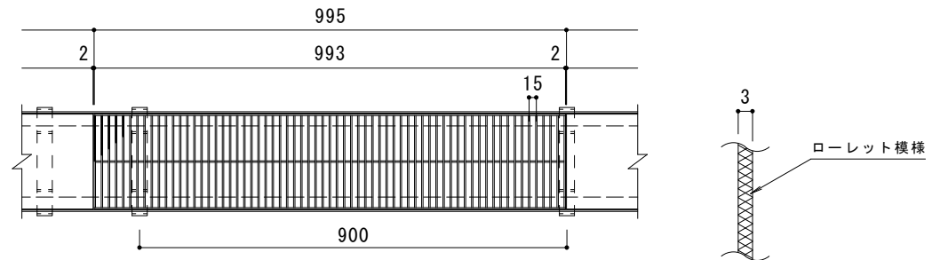
メインバー表面 S = 1 : 1
