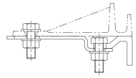
A-A断面図 S=1:3
