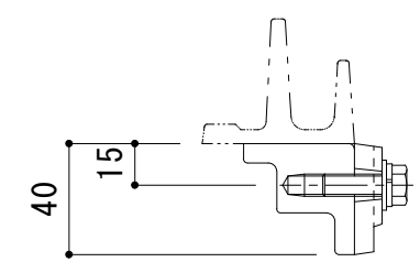
B-B断面図 S=1:3
