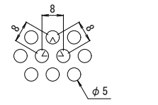
バスケット穴詳細図 S=1:1
