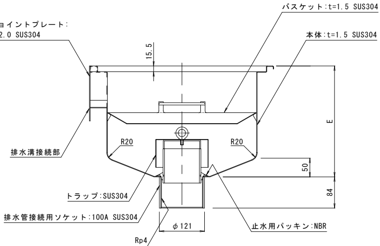
A-A断面図
