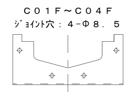
ジョイント穴詳細
