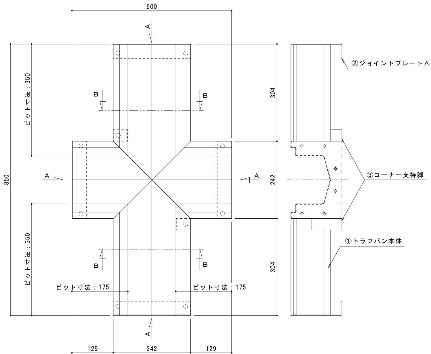
寸法表 [mm]
