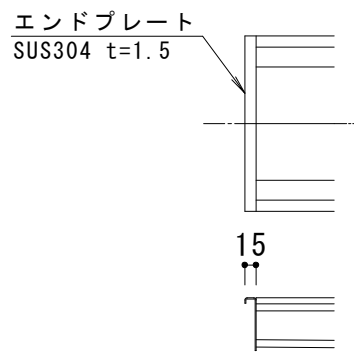
水上側エンドプレート S=1:10
