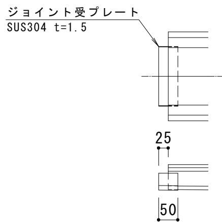
ジョイント受プレート S=1:10
