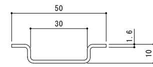
補強材詳細図 S=1:1
