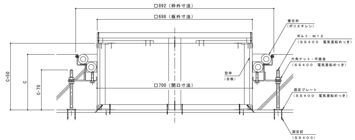
打込金具 納まり図 S=1:5
