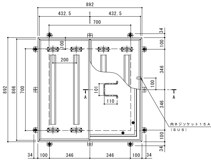
平面詳細図 S=1:10
