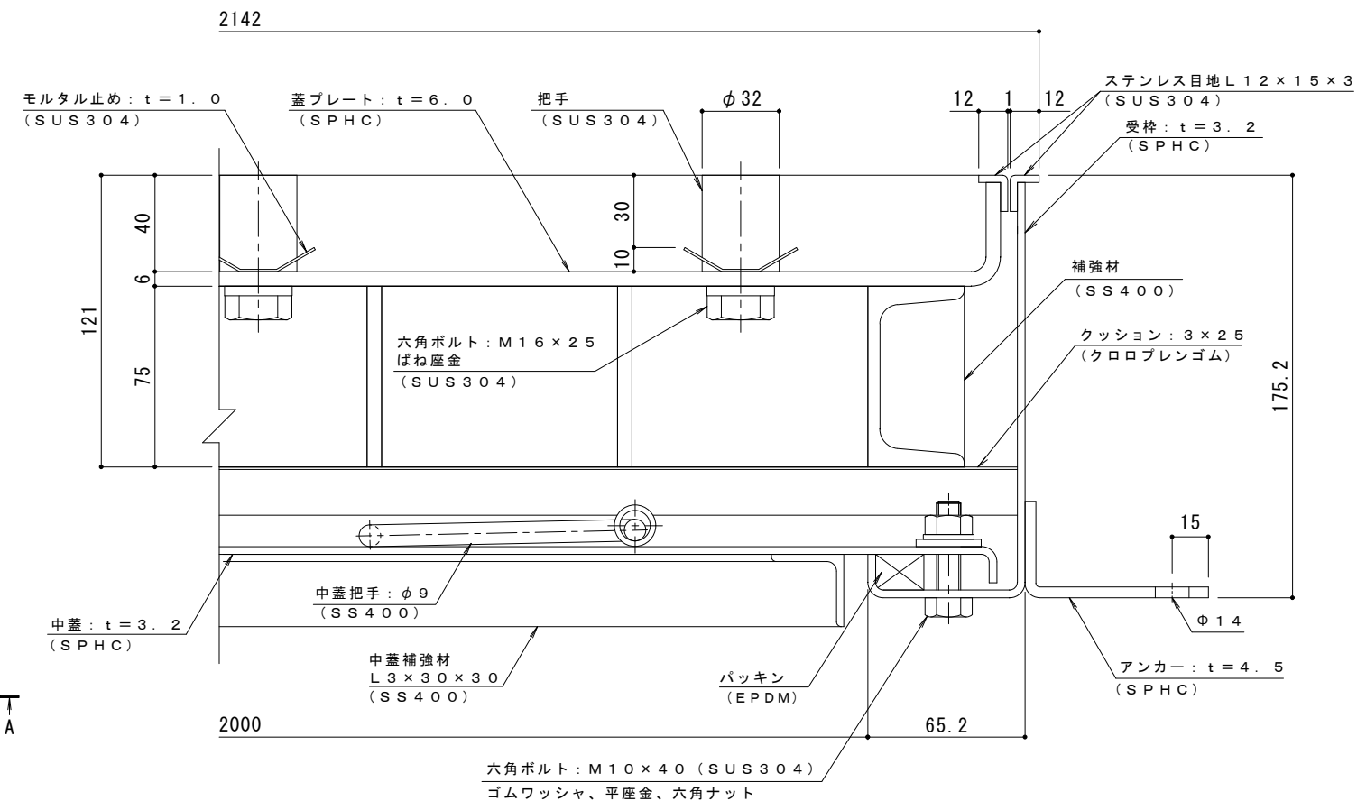
A-A断面詳細図 S = 1 : 2
