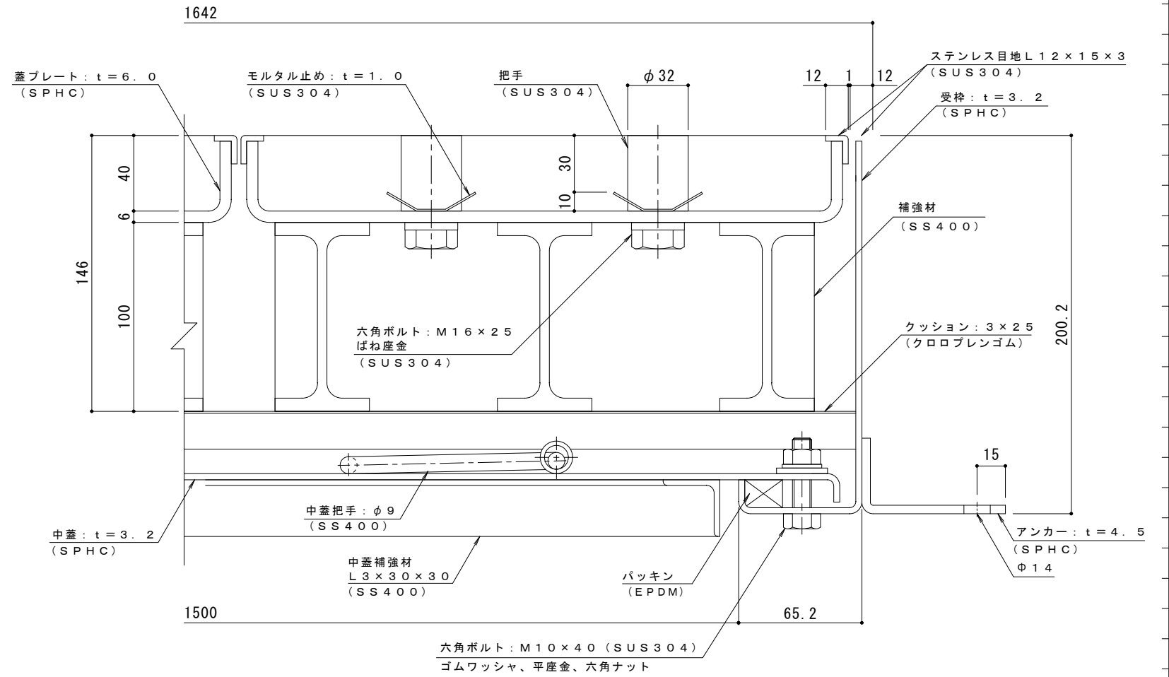
A-A断面詳細図 S = 1 : 2
