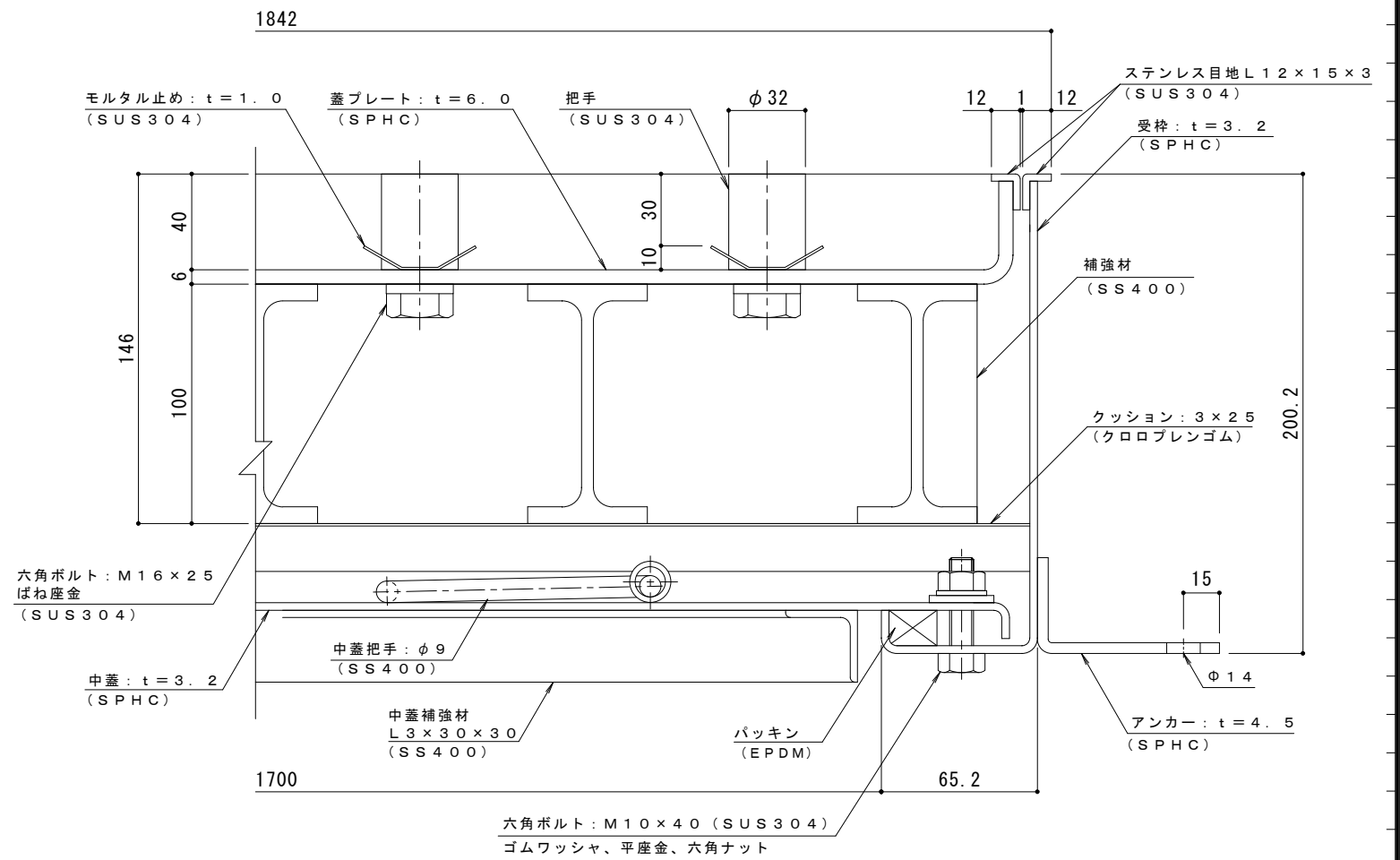
A-A断面詳細図 S = 1 : 2
