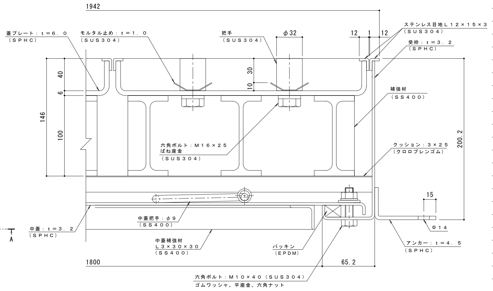
A-A断面詳細図 S = 1 : 2
