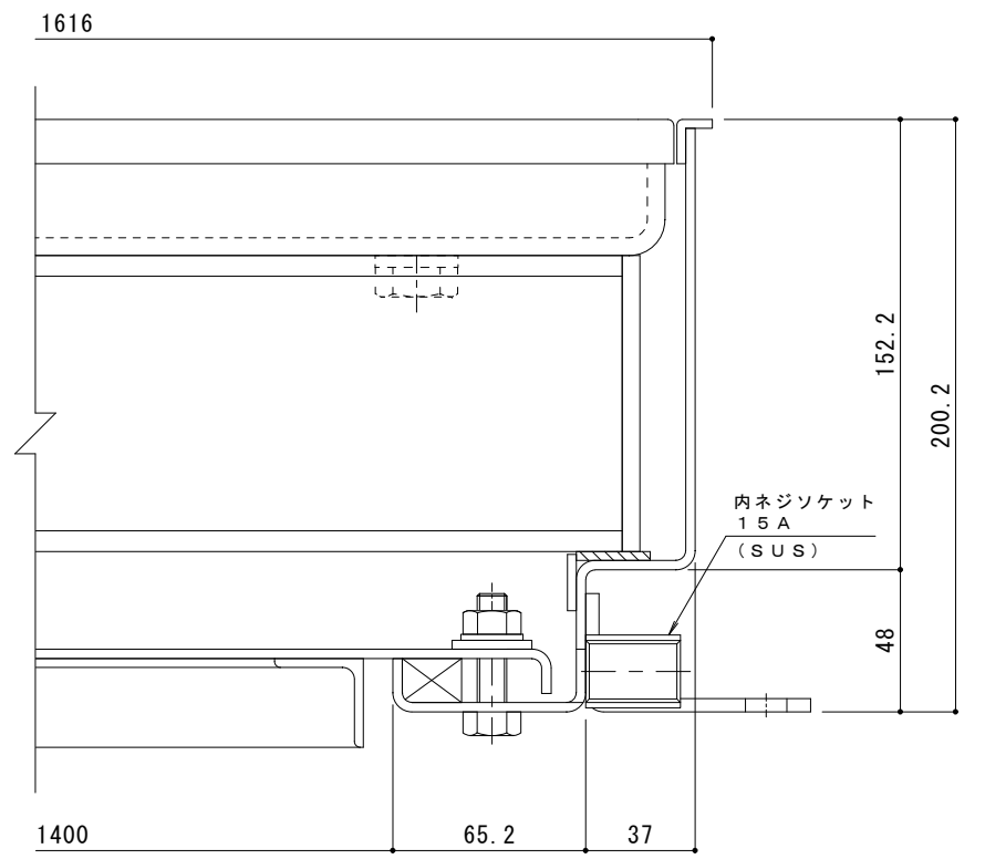
B-B断面詳細図 S = 1 : 2
